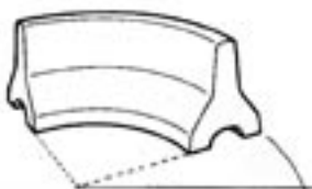
CITYBLOC oblouk 100 CTB 504 44/50/R100 cm 90° 320 kg
